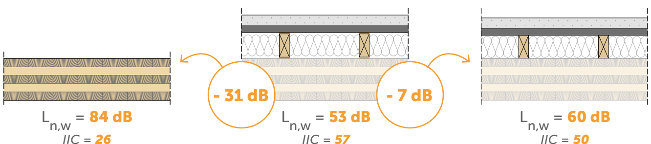
Einbau des Trockenbausystems mit PIANO
